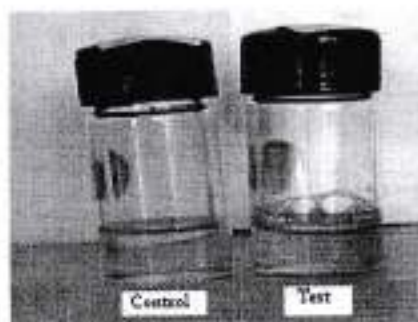
Photoplate 3:- Csaky's Assay
